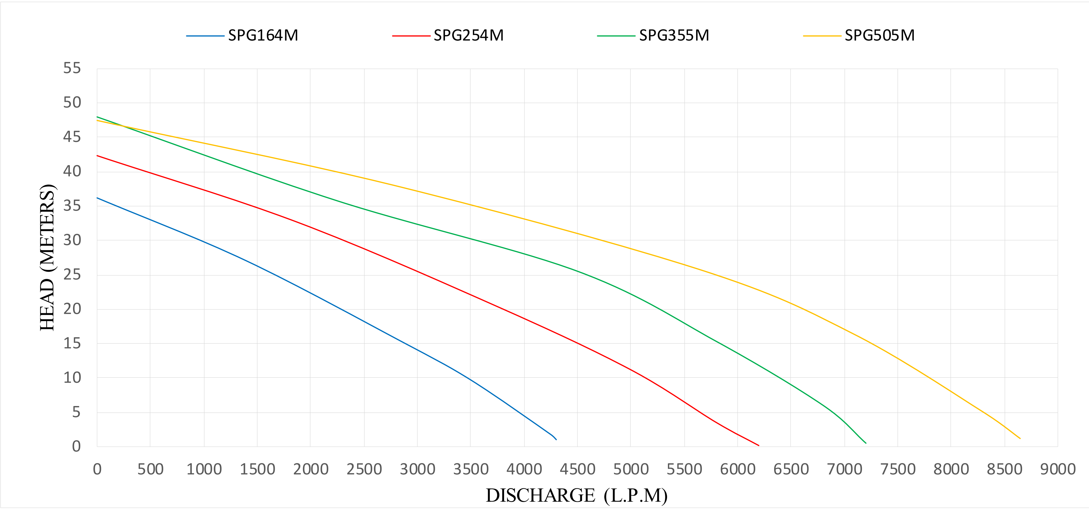
16 to 50 HP (Medium Head)
